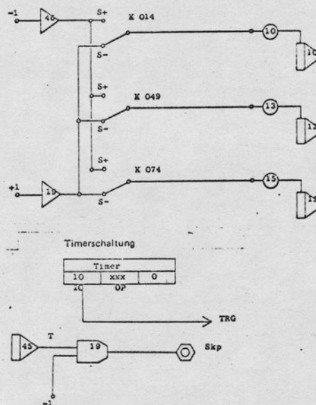
Bild 3. Aufbringen der berechneten Anfangsbedingungen
