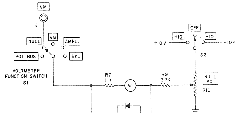
(d) NULL POSITION
