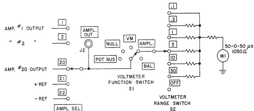
(b) AMPL POSITION
