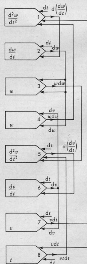
Bild 13. Rechenschaltung für Gl. (10).
