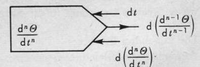
Bild 9. Integrator.
